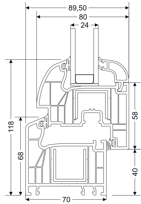
PRO7006 Kasa (6 Odacıklı) - Damlalıklı Kanat Kesit Detayı
