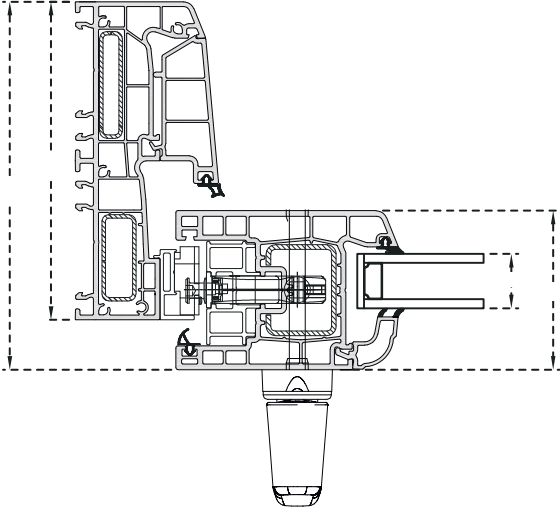
Kasa-Kanat Kapalı Pozisyon
