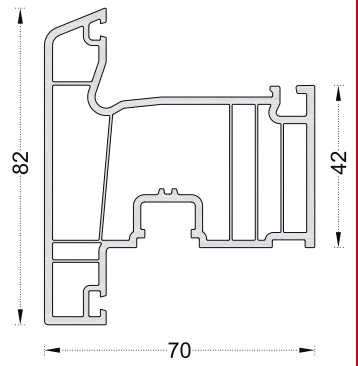
PRO722 T Kanat
