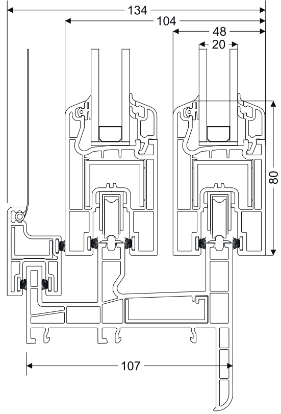
Pervazlı, Sineklikli Çift Sürme Kasa - Sürme Kanat - Sürme Sineklik Kanat Kesit Detayı
