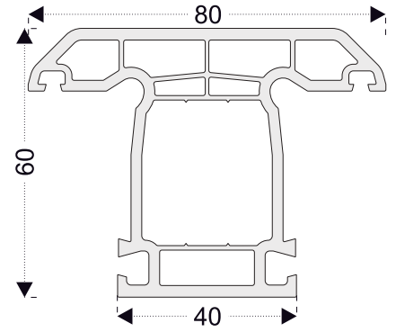
PRO03 Orta Kayıt
