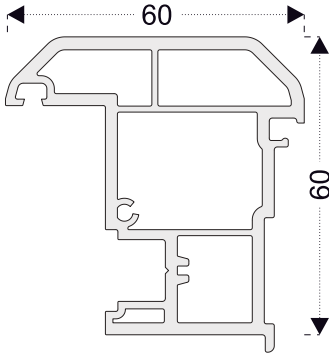
PRO12 Hareketli Orta Kayıt
