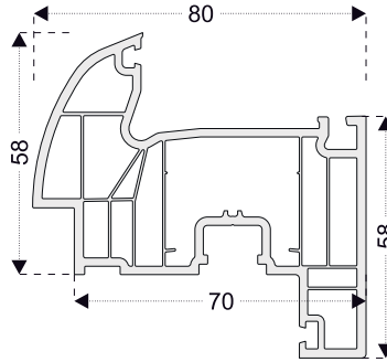
PRO724 Damlalıklı Kanat (7 Odacıklı)
