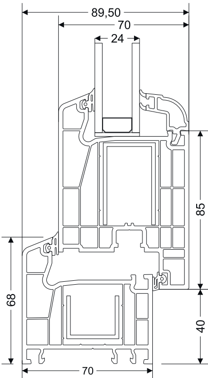
Kasa - Z Kapı Kanat Kesit Detayı
