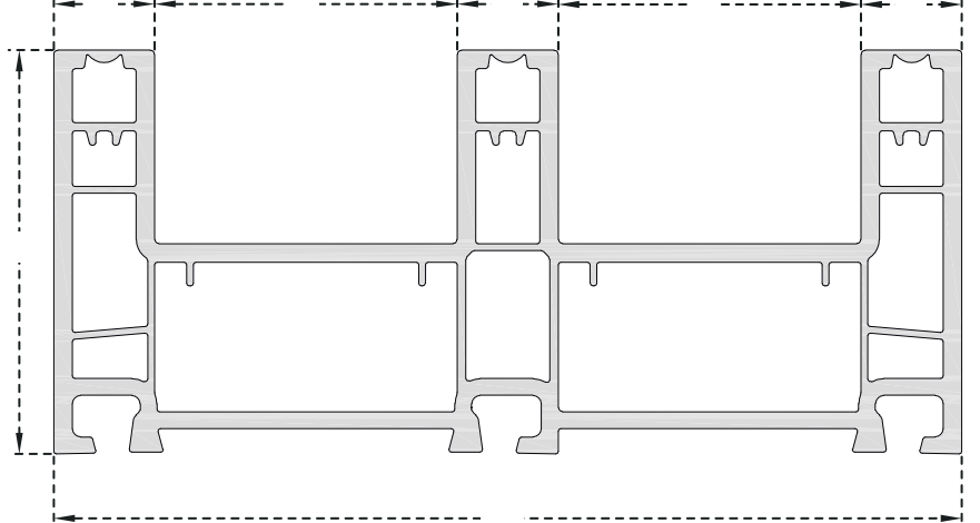
PRO601 60mm Üçlü Sürme Kasa
