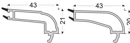
PRO700 4-6 mm Cam Çıtası
