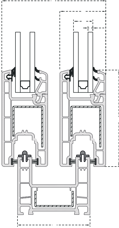
Sürme Kasa - Sürme Kanat (80 mm) Kesit Detayı
