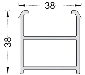
PRO1007 Montaj Yükseltme Profili
