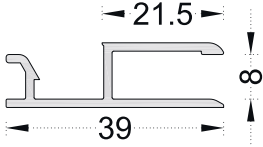
PRO31A Pervaz Adaptör Profili
