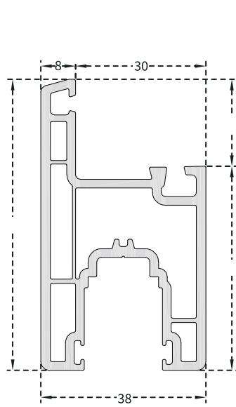
PRO604 60mm Sürme Kanat (67 mm)
