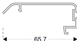
PRO43 Tek Sürme Kasa Kapama (Alüm.)
