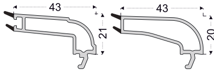
PRO720 Kasa (6 Odacıklı)
