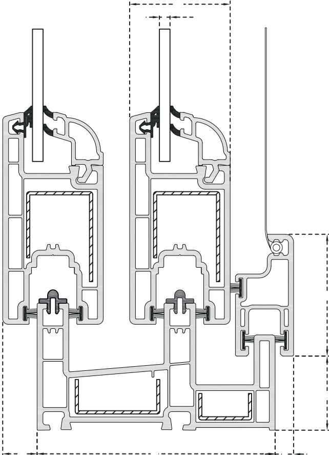
Sürme Sineklikli Kasa (Sineklik İçte) - Sürme Kanat Kesit Detayı
