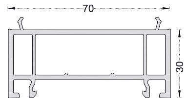
PRO1008 30mm Yükseltme (70 mm Serisi)
