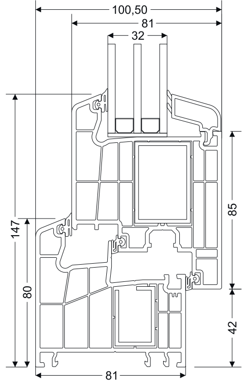
Kasa - Z Kapı Kanat Kesit Detayı
