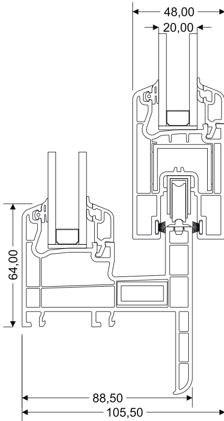
Pervazlı, Tek Sürme Kasa, Sürme Kanat Kesit Detayı
