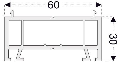
PRO14 30 mm Yükseltme (60 mm Serisi)
