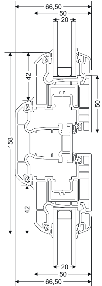
Kanat - Orta Kayıt - Kanat Kesit Detayı
