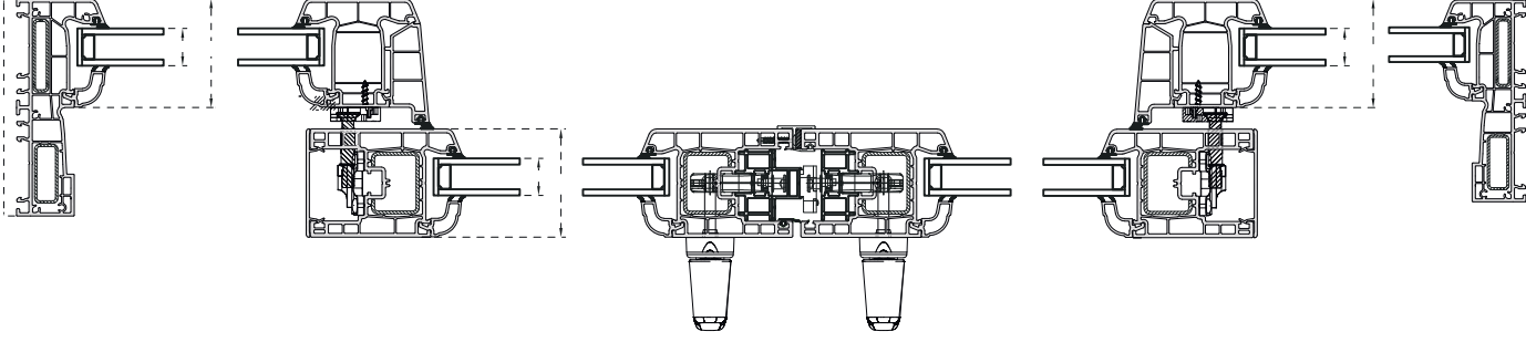
Çift Kanatlı Kapalı Pozisyon
