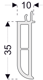
PRO39 Tırnaklı Pervaz (70mm Seri)
