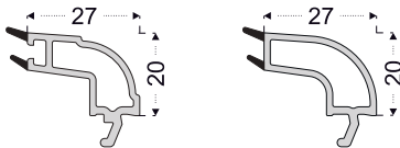
PRO701 20-22 mm Çift Cam Çita
