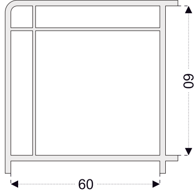
PRO36 Kutu - 60x60mm (60mm Seri)
