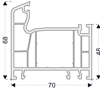
PRO710 Kasa - 48mm
