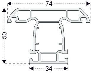
PRO533 Orta Kayıt
