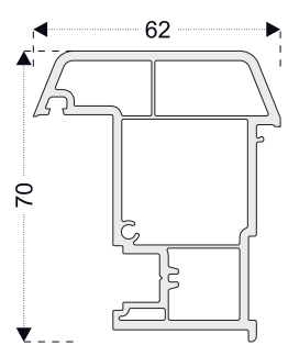
PRO717 Hareketli Orta Kayıt
