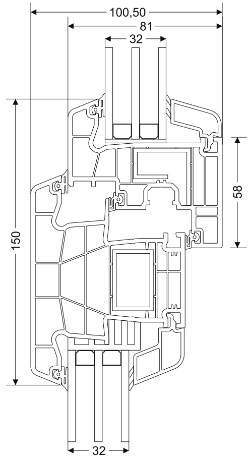
Kanat - Orta Kayıt - Sabit
