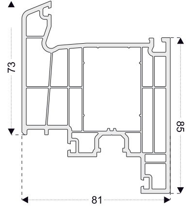
PRO8631 Z Kapı Kanat
