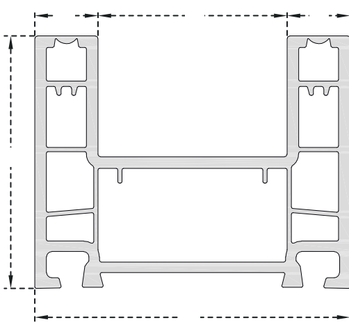
PRO600 60mm Çift Ray Sürme Kasa
