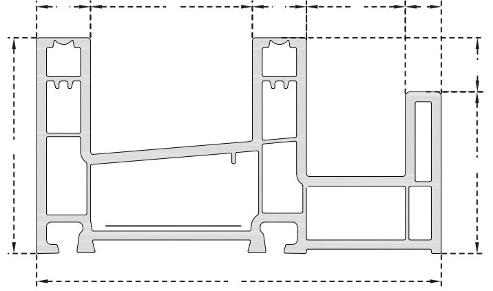
PRO603 60mm Sürme Sineklikli Kasa (Sineklik İçte)
