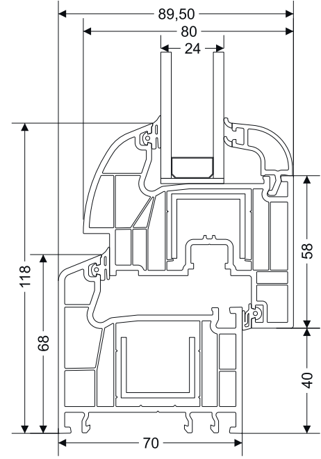
Kasa - Damlalıklı Kanat Kesit Detayı
