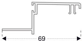
PRO28 Çift Sürme Kasa Kapama (Alüm.)
