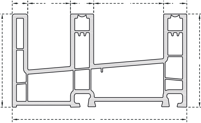
PRO602 60mm Sürme Sineklikli Kasa (Sineklik Dışta)
