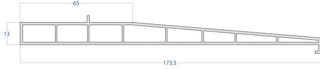
PRO75 Denizlik Profili
