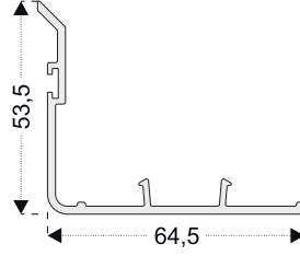
PRO25 ** PRO24 için Sürme Kanat Adaptörü
