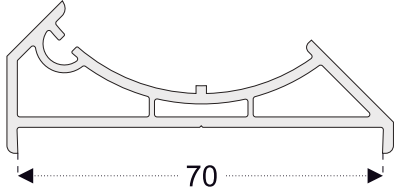
PRO331 Köşe Dönüş Adaptörü - 70mm
