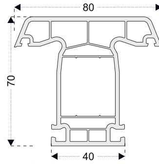
PRO713 Orta Kayıt
