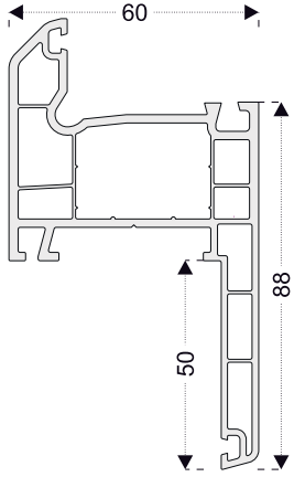
PRO582 Pervazlı Kasa
