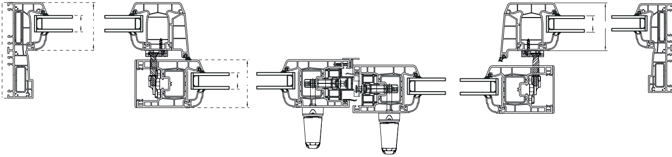
Çift Kanat Sürme Pozisyon
