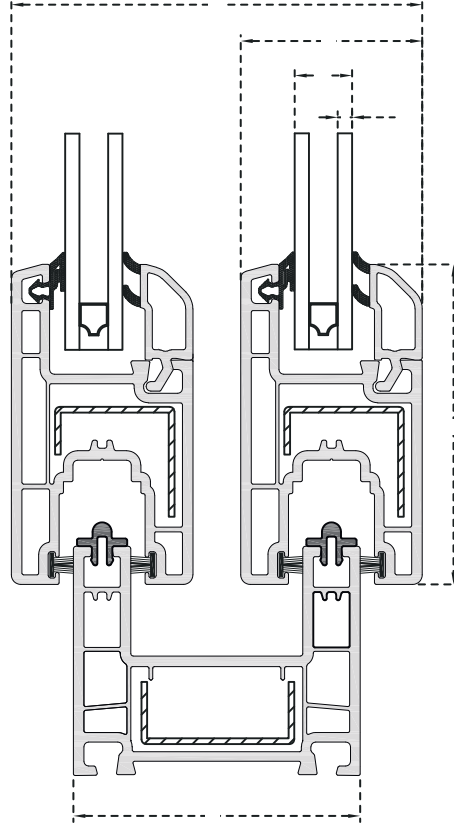
Sürme Kasa - Sürme Kanat (67 mm) Kesit Detayı
