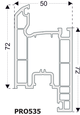
PRO535 Z Kapı Kanat
