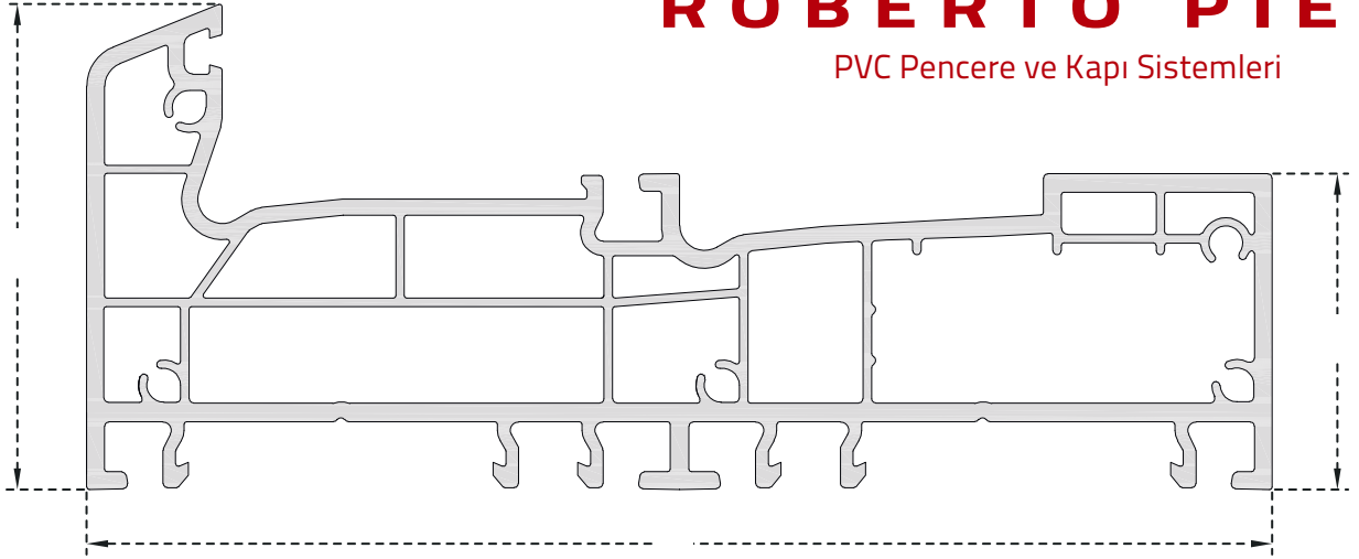
PRO1400 Sürme Kasa
