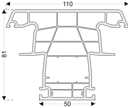
PRO8621 Kasa Orta Kayıt Profili
