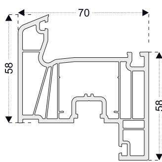
PRO723 Kanat (6 Odacıklı)
