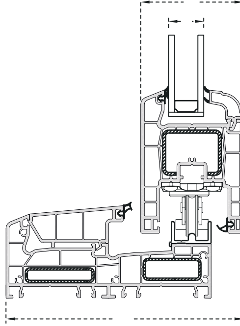
Kasa-Kanat Sürme Pozisyon
