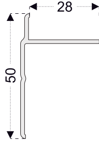
PRO35 T Pervaz (60mm Seri)
