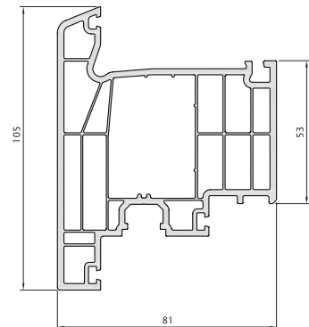
PRO8632 8106 Dışa Açılan Kapı Kanat
