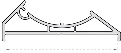
PRO8638 Köşe Dönüş Adaptörü - 81 mm
