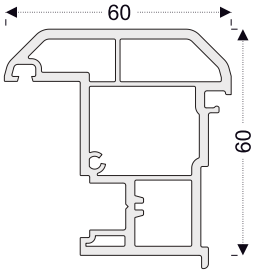
PRO12 Hareketli Orta Kayıt
