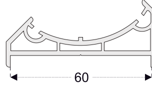
PRO33 Köşe Dönüş Adaptörü - 60mm
