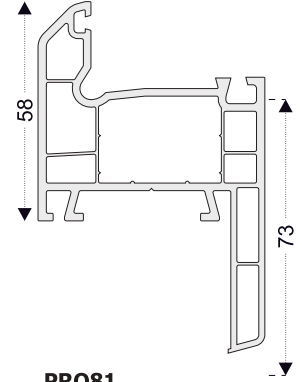
PRO81 Pervazlı Kasa
