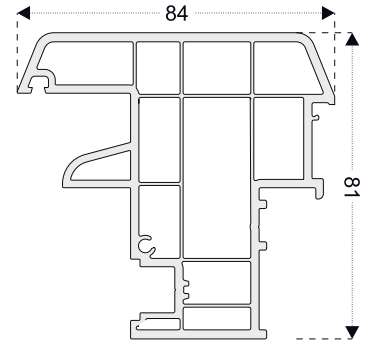
PRO8622 Hareketli Orta Kayıt
