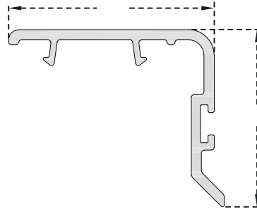
PRO606 60mm Sürme Kanat Adaptörü
