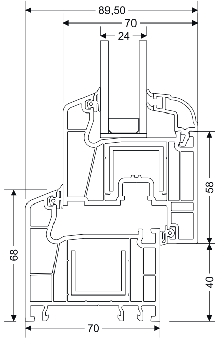
Kasa 48mm - Kanat Kesit Detayı
