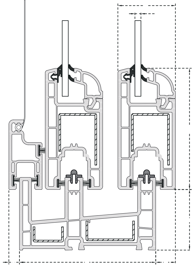
Sürme Sineklikli Kasa (Sineklik Dışta) - Sürme Kanat Kesit Detayı
