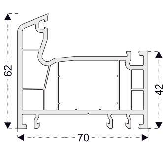
PRO711 Kasa - 42mm
