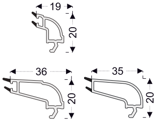
PRO05 20-22 mm Çift Cam Çita
