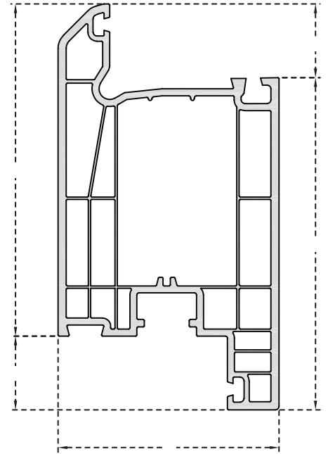
PRO17 6004 Kapı Kanat
