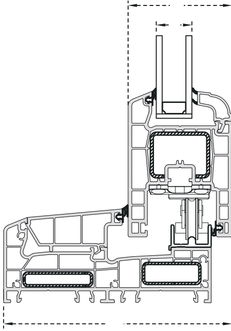
Kasa-Kanat Kapalı Pozisyon
