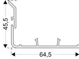
PRO22 ** PRO21 için Sürme Kanat Adaptörü
