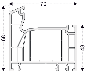
PRO720 Kasa (6 Odacıklı)
