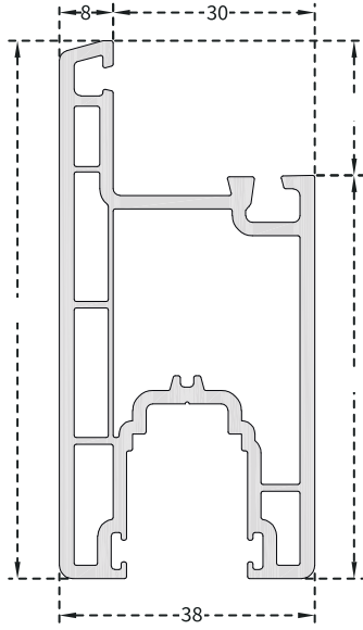
PRO605 60mm Sürme Kanat (80 mm)
