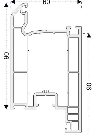
PRO04 Z Kapı Kanat
