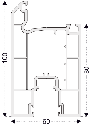
PRO24 Sürme Kanat
