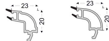
PRO702 24-26 mm Çift Cam Çita
