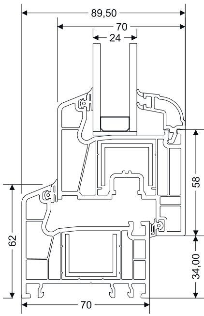
Kasa 42mm - Kanat Kesit Detayı
