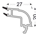
PRO700 4-6 mm Cam Çıtası
