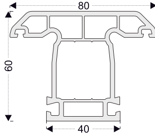
PRO53 Orta Kayıt
