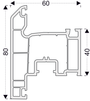
PRO521 T Kanat
