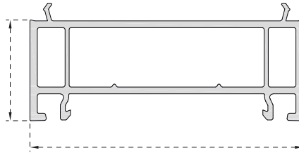
PRO8639 30 mm Yükseltme (81 mm Serisi)
