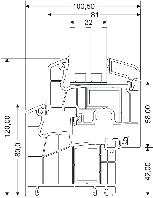
Kasa - Kanat Kesit Detayı
