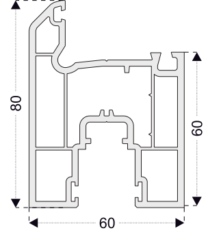
PRO21 Sürme Kanat
