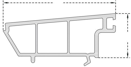
PRO1402 Sürme Kasa Kapama
