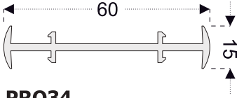
PRO34 Bağ - 60mm
