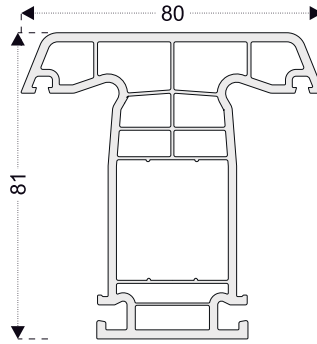
PRO8623 Kanat Orta Kayıt Profili
