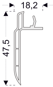
PRO38 Tırnaklı Pervaz (60mm Seri)
