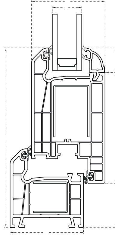
Kasa - İçe Açılan Kapı Kanat Kesit Detayı
