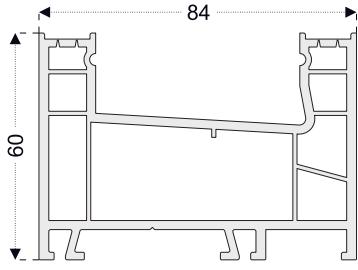
PRO20 Çift Sürme Kasa
