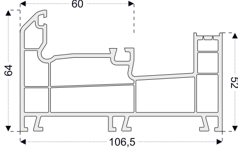
PRO23 Tek Sürme Kasa
